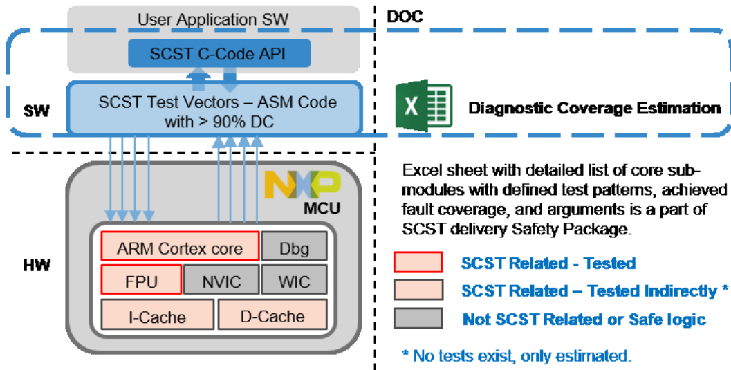
图 1. 恩智浦的 SCST 库内容示例
